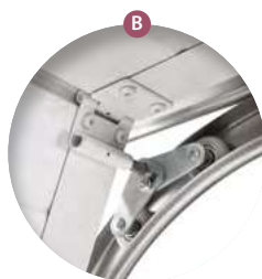
Galets duo flex sur charnières anticorrosion laquées blanches, robustes et discrètes
