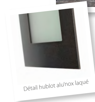
Rectangle alu'nox laqué - 4 tailles : 511 x 321 / 600 x 200 / 1100 x 200 / 1600 x 200 mm
